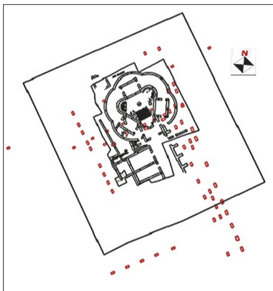
Fig. 9 – Evidenze archeologiche (in rosso) intercettate dalle tomografie geoelettriche.
