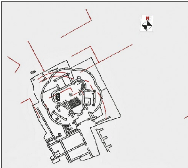
Fig. 11 – Anomalie (in rosso) risultanti dalle prospezioni magnetometriche.
